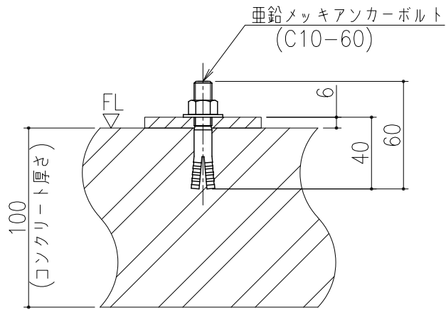
アンカーボルト取付図 (S=1/3)
